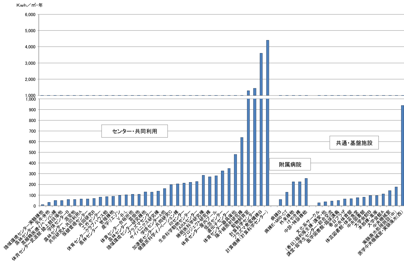
図2-2 単位面積当たり電気使用量(センター・共同利用・附属病院・共通・基盤施設)
